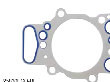
CABEÇOTE (C/ ANÉIS INJETADOS) 124 400EV/420 ELETRÔNICO
