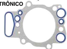
CABEÇOTE (C/ ANÉIS INJETADOS) 124 400EV/420 ELETRÔNICO
