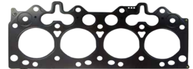
JUNTA DO CABEÇOTE 1,59mm
