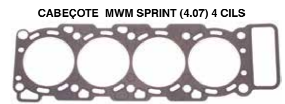
CABEÇOTE MWM SPRINT (4.07) 4 CILS 71002ECO-SC N° ORIG.9.407.0854.8074
